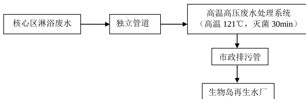
图 5.1-3 核心区淋浴废水处理工艺流程
