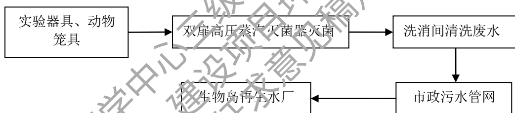
图 5.1-2 洗消间废水处理工艺流程
