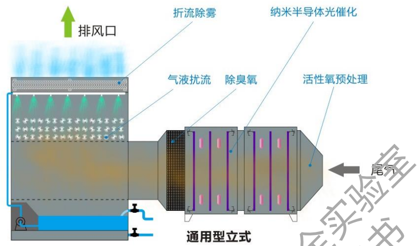
图 5.2-7 一体扰流喷淋除臭设备结构示意图
