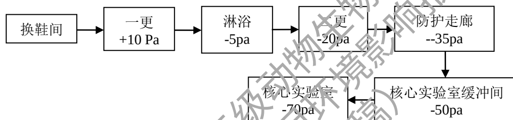
图 2.1-13 实验室各单元相对压力梯度图
