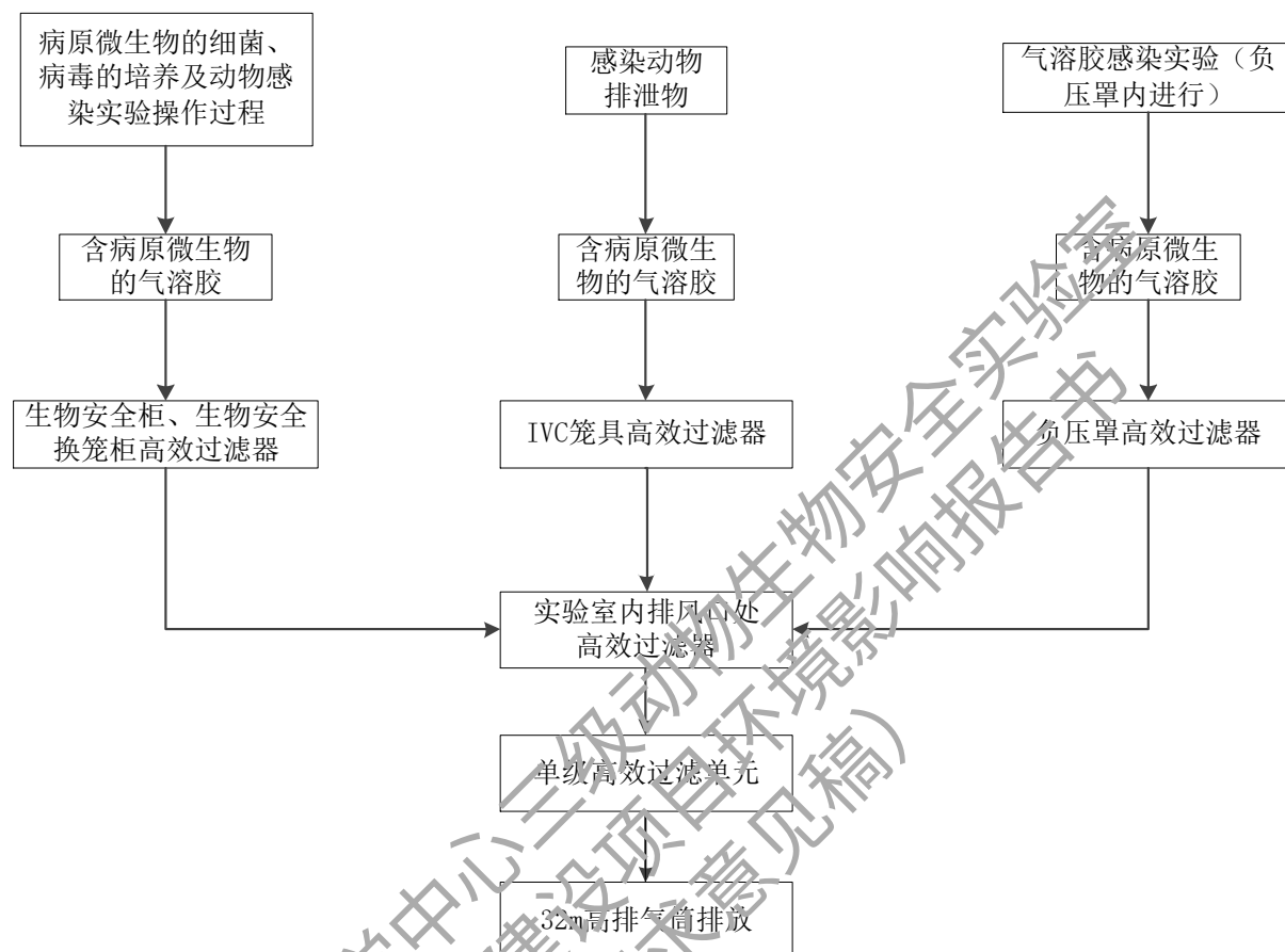
图 5.2-1 含病原微生物的气溶胶防治措施工艺流程图
