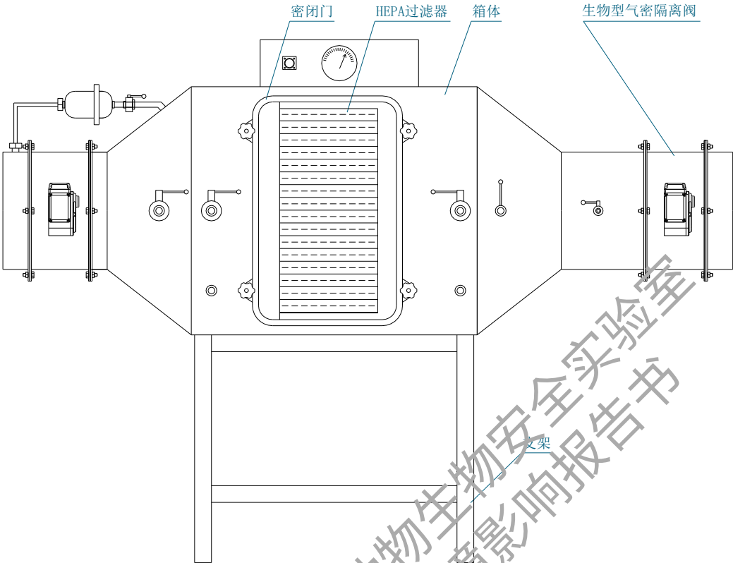
图 5.2-3（a） 实验室高效过滤单元结构示意图
