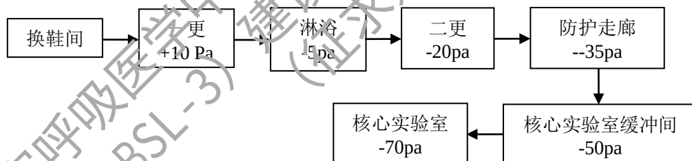
图 6.6-1 实验室各单元相对压力梯度图
